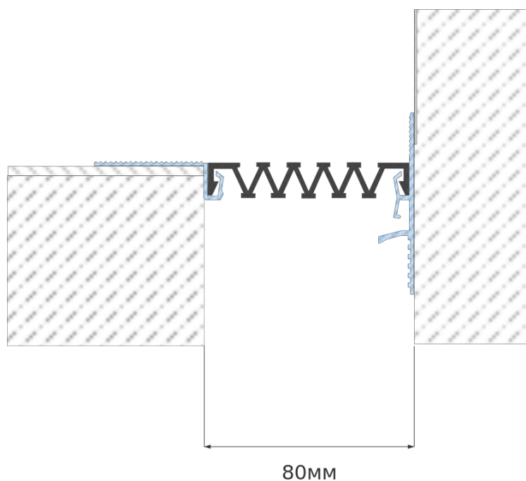
ЧЕРТЁЖ
