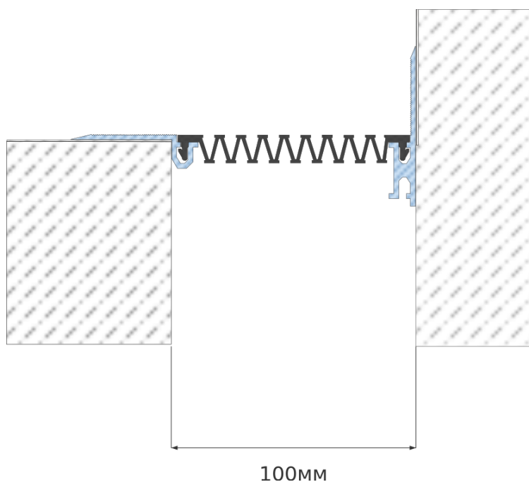
ЧЕРТЁЖ
