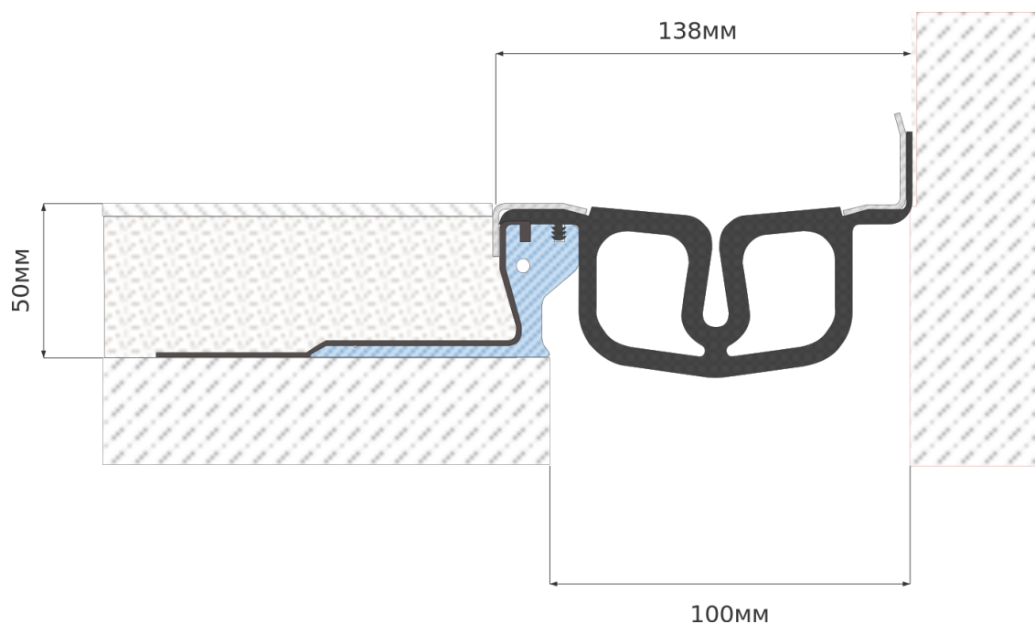
ЧЕРТЁЖ
