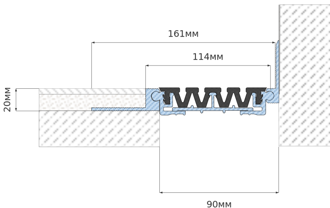
ЧЕРТЁЖ
