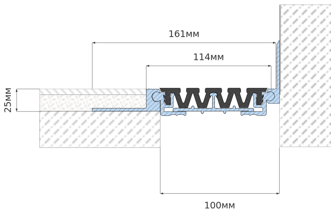
ЧЕРТЁЖ
