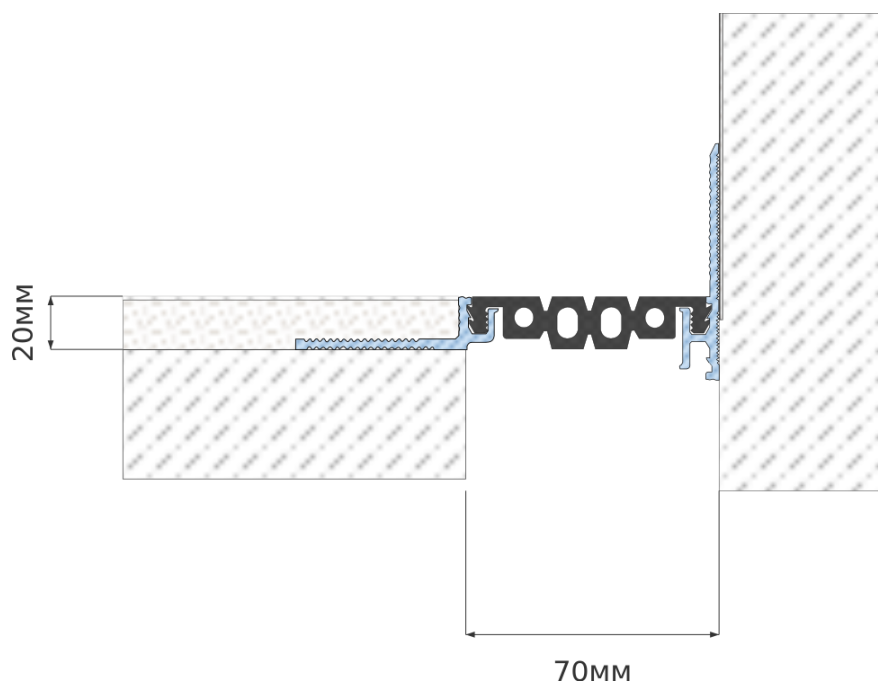
ЧЕРТЁЖ
