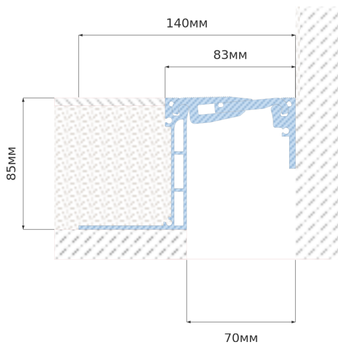
ЧЕРТЁЖ
