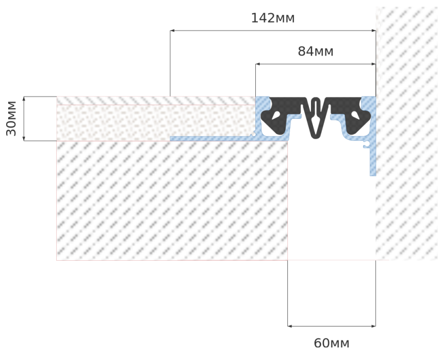
ЧЕРТЁЖ
