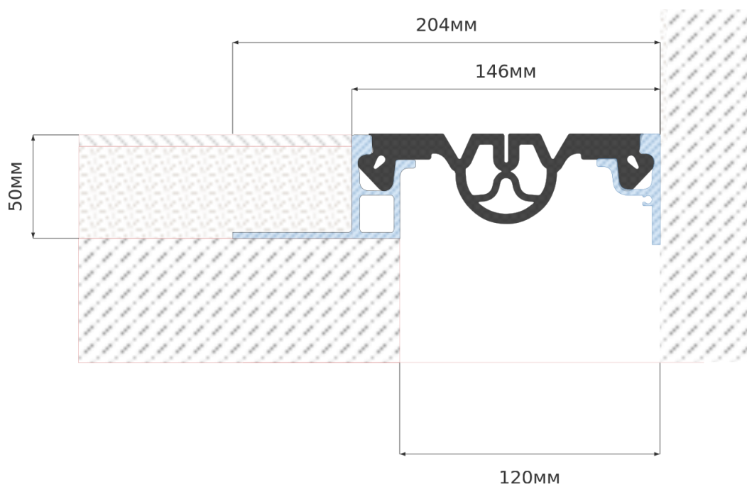
ЧЕРТЁЖ
